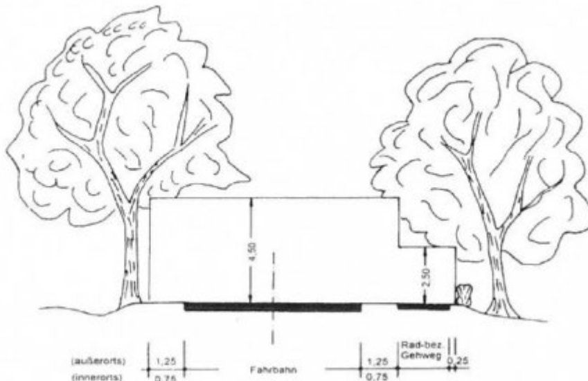
Lichtraumprofil
